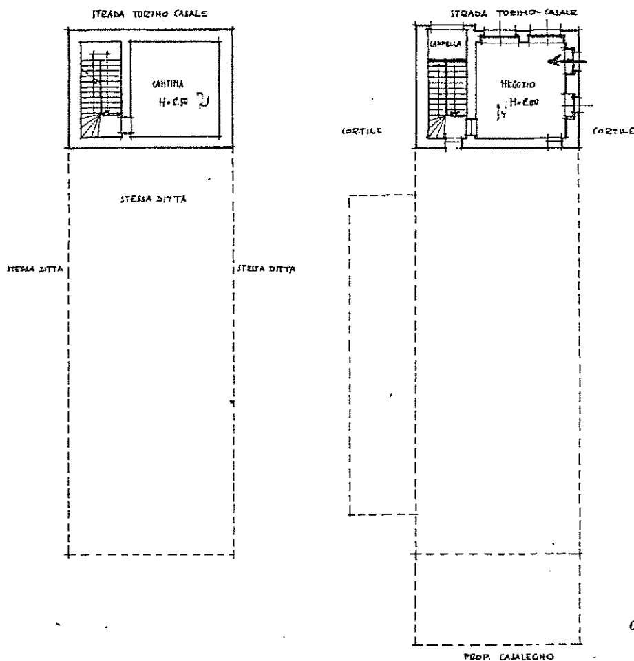
PIANTA PIANO CANTINATO
